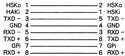
mini DIN 8pin male
